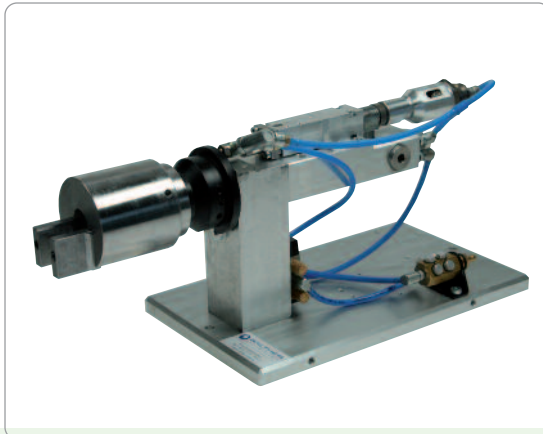
Dispositivo de engrasado de mesa para componentes de plástico
